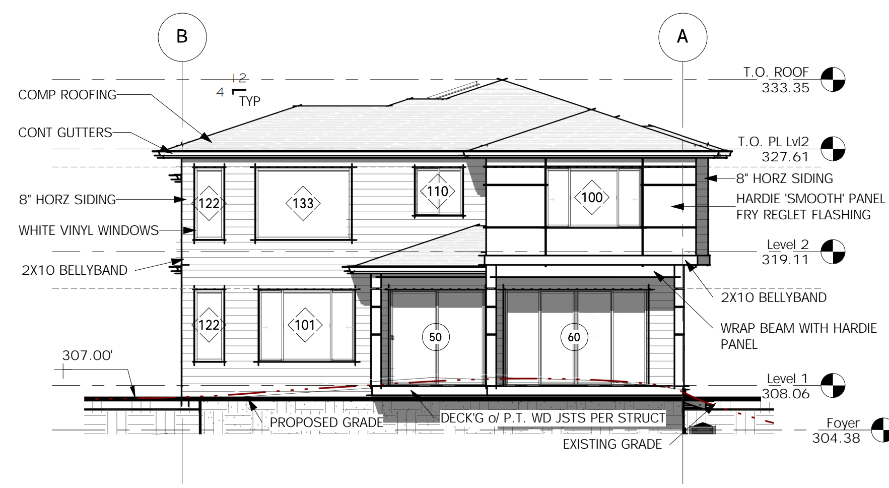
2 EAST ELEVATION SCALE: 1/8" = 1'-0"
