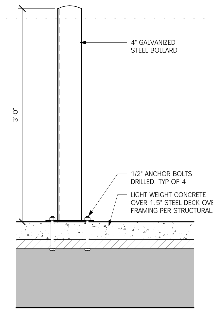
4 BOLLARD DETAIL SCALE: 1 1/2" = 1'-0"
