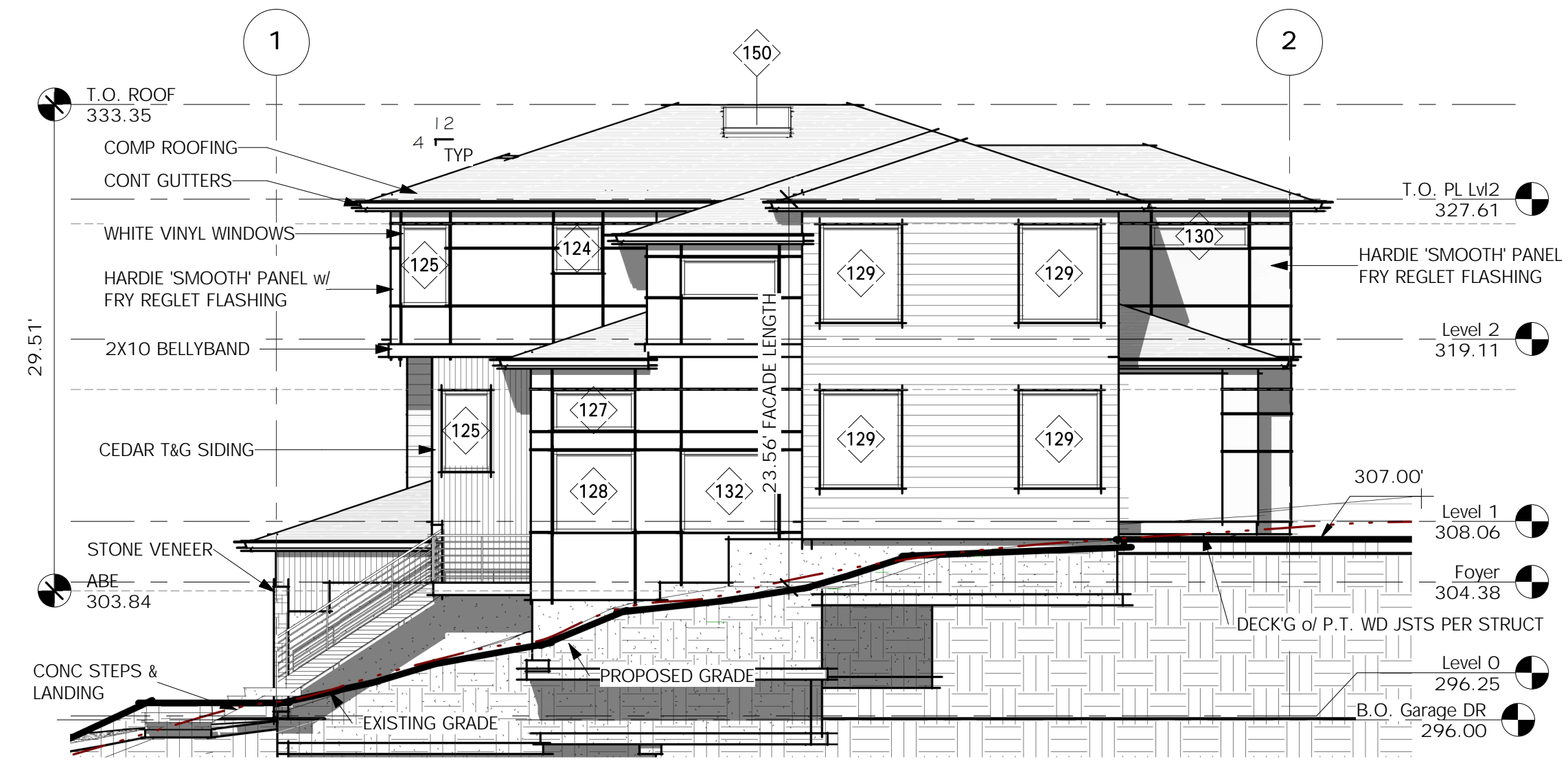
4 SOUTH ELEVATION SCALE: 1/8" = 1'-0"
